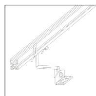
Fixage à levier pour toit incliné
